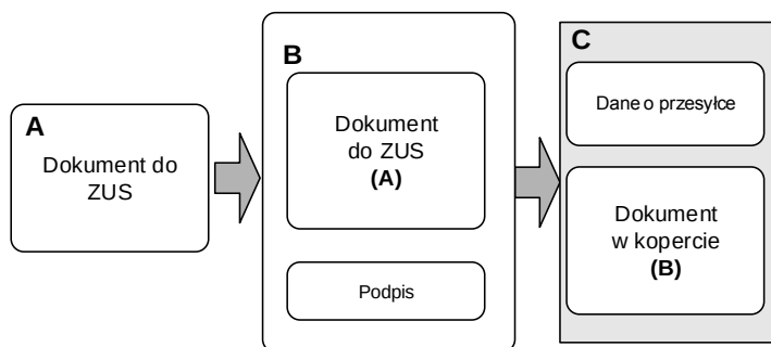
Rysunek 37 Schemat tworzenia przesyłki z ZUS (komunikat INawsUslugi_PobierzPotwierdzenie_OutputMessage )
