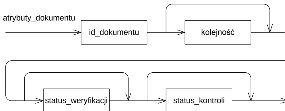
Rysunek 14 Atrybuty dokumentu
